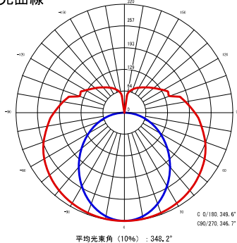
配光曲線
