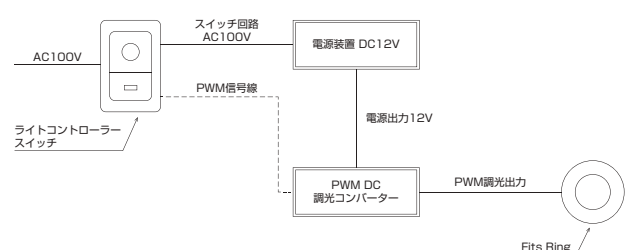
PWM 調光結線例
