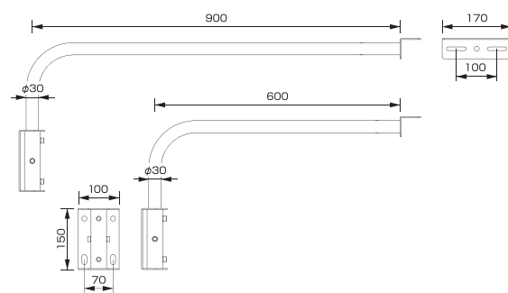
■専用アーム寸法図
